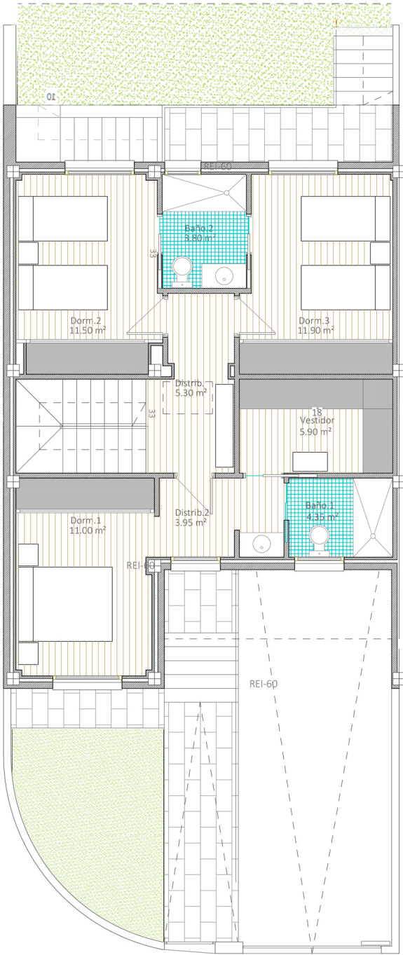
PL. PRIMERA
